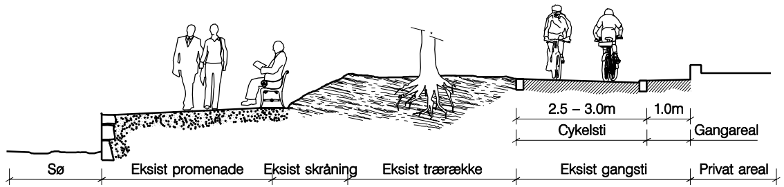
Principsnit i strækning type A
