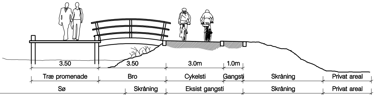
Principsnit i strækning type C1
