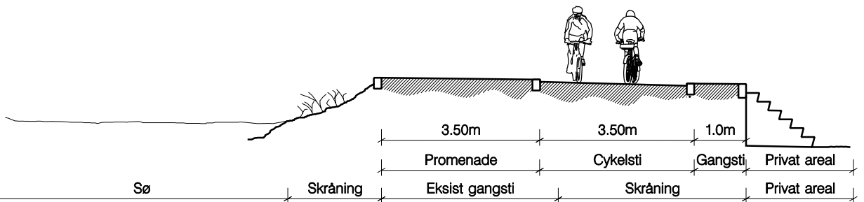
Principsnit i strækning type C2
